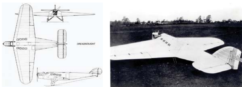
Рисунок 7. Опытный образец почтово-пассажирского самолета Westland Dreadnought (модель 1920–1924 гг.) с крылом Н.С. Воеводского
